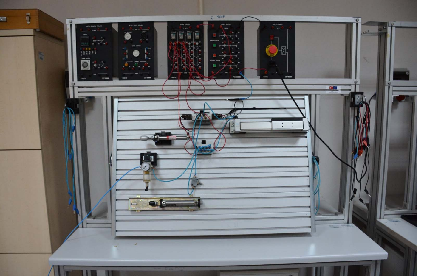
PNÖMATİK VE ELEKTROPNÖMATİK DENEY SETİ
